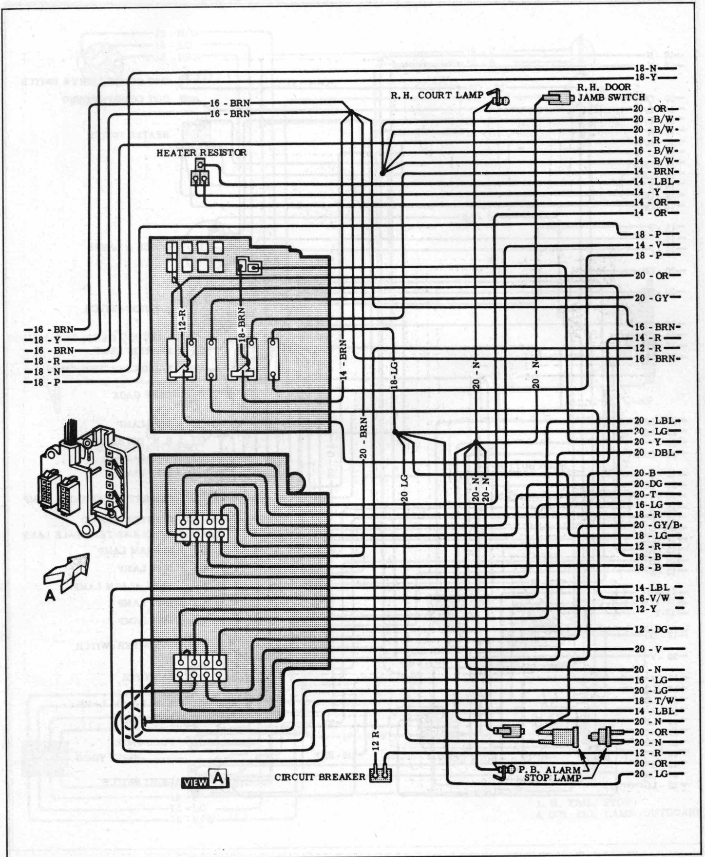
Fig. 41b—Fuse Panel Wiring
