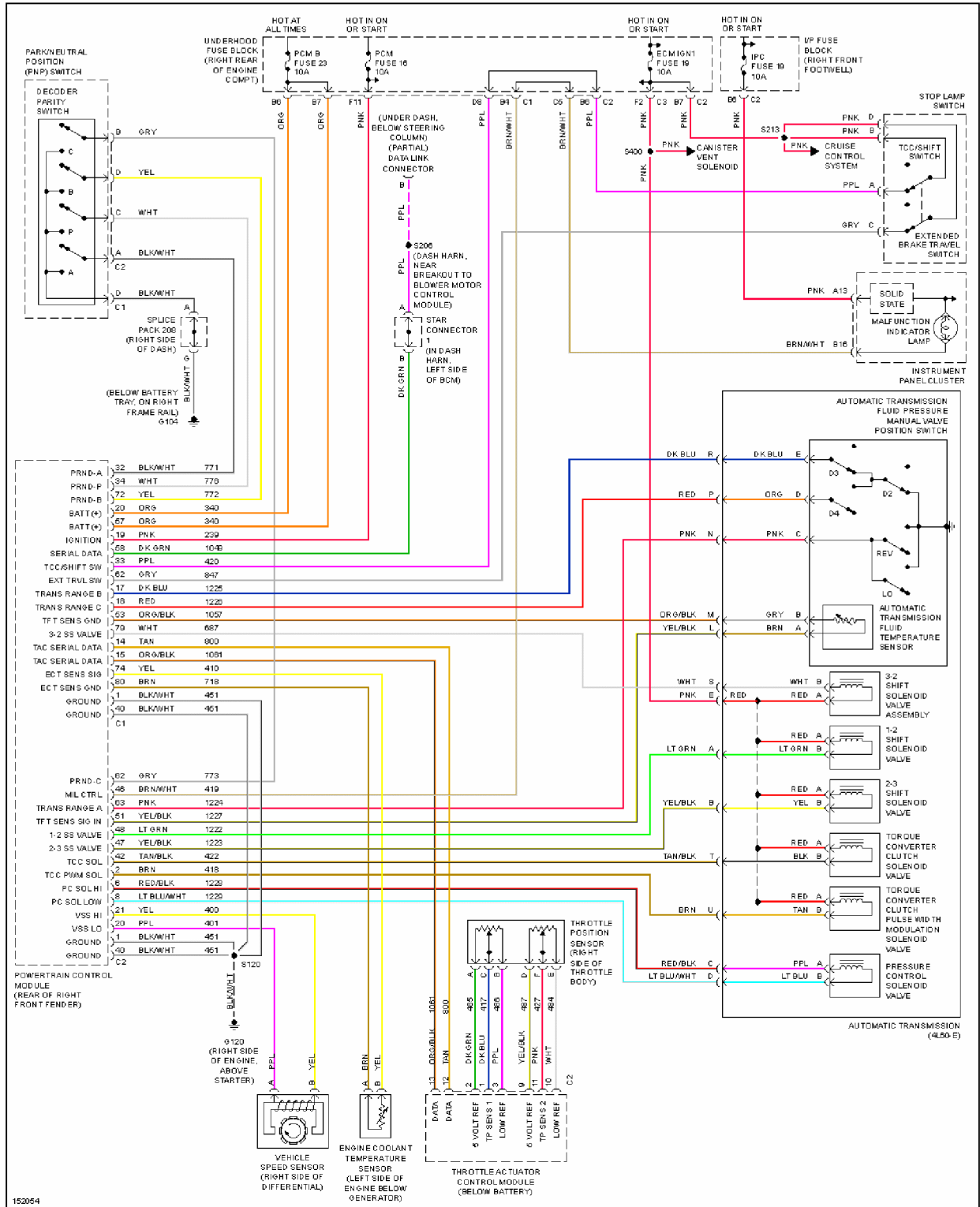
Fig. 46: 5.7L VIN G, A/T Circuit
