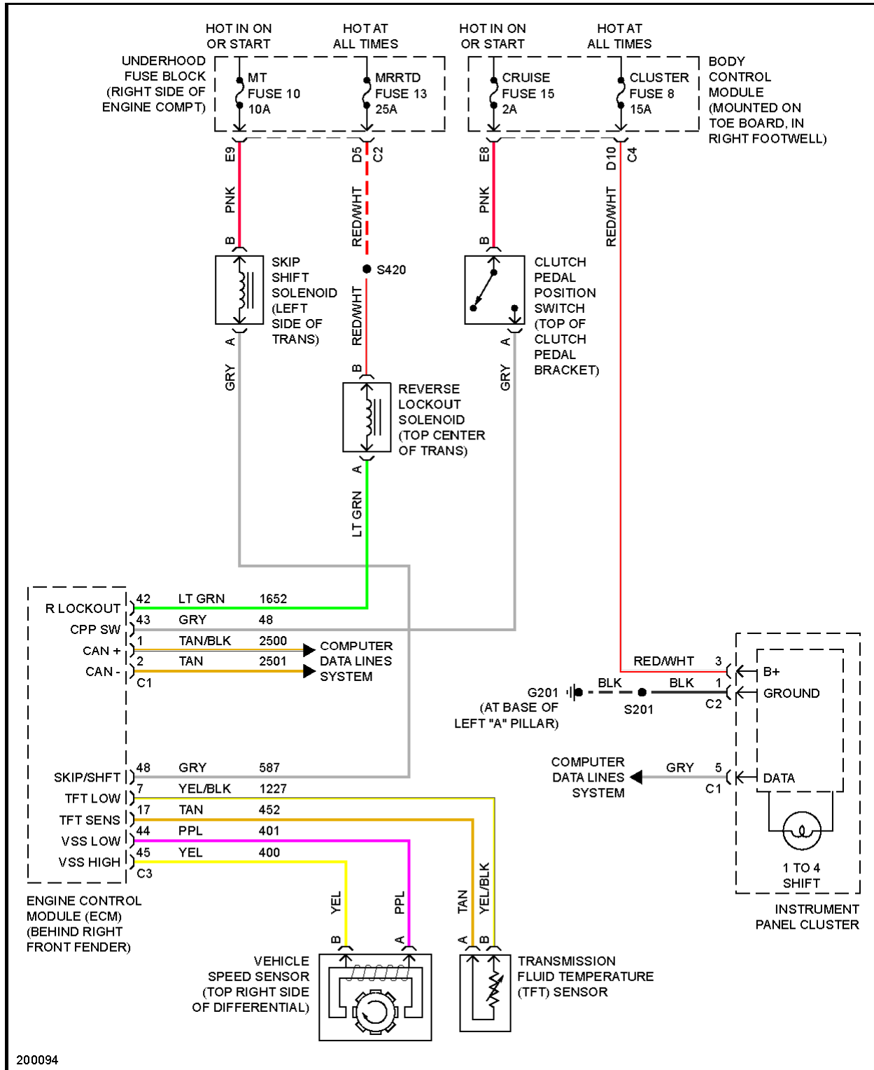
Fig. 68: M/T Circuit
